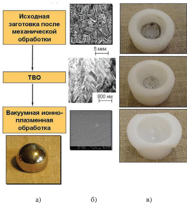
Рис. 3. Инновационная комплексная технология получения изделий из титанового сплава ВТ6: технологическая схема изготовления головки эндопротеза тазобедренного сустава (а); изменение объемной структуры и состояние поверхности головки (б); результаты ресурсных испытаний головки в разных структурных состояниях в паре со сверхвысокомолекулярным полиэтиленом (в)
