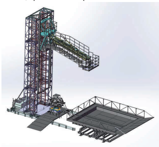
Рис. 2. Стенд обработки мягкой посадки лунных космических аппаратов
